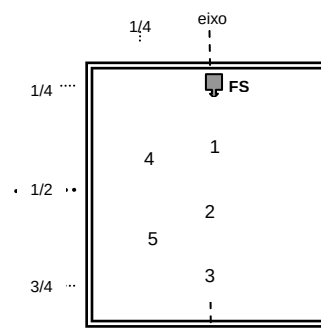
Figura 2.37 – Localização dos pontos de medição e da fonte sonora (FS) nas salas de desporto para a determinação do parâmetro RASTI (Inteligibilidade da Palavra).
