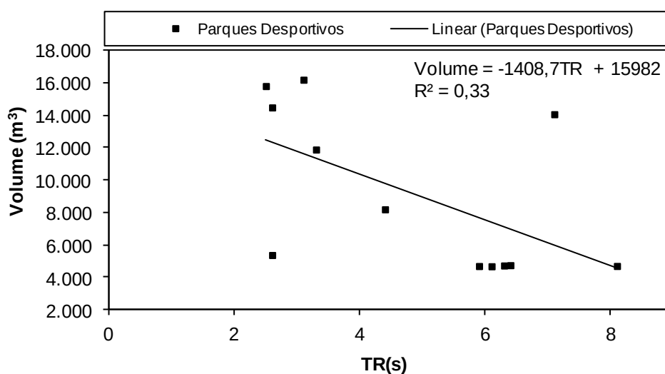
Figura 3.82 - Melhor correlação entre os valores médios do Volume (m³) e os valores médios do TR (s) nos 14 PDE.
